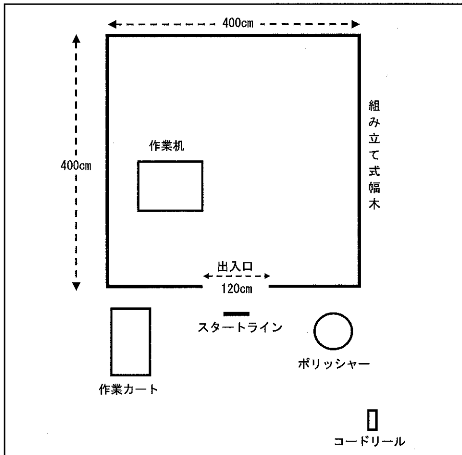
<標準配置図>
